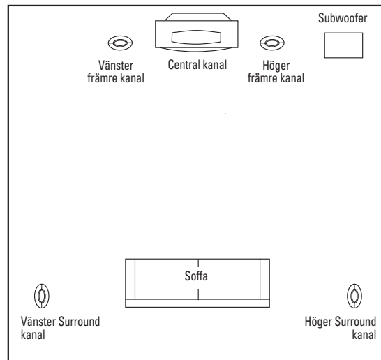
Figur 1. I den här visningen ovanifrån av en typisk installation används satellithögtalarna för att återge ljud för den främre kanalen och surroundkanalen. Centralkanalen återger ljud och dialog. Den nätanslutna subwoofern ger bas för effekter och musik.
