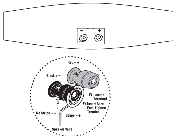
Figur 5. Alla terminaler på högtalarna, kan anslutas på flera olika sätt, banan, spade eller som här direkt med kabeln.
