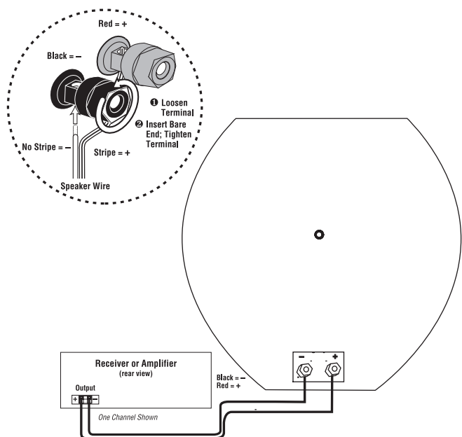
Figur 4. Kopplingsdiagram visar polaritetskopplingar för en kanal i ett hemmabiosystem.
